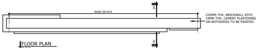
FLOOR PLAN N.T.S
