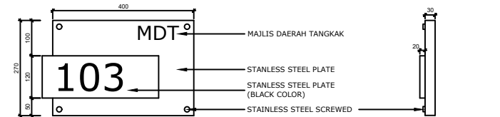
DETAIL SIGNAGE N.T.S
