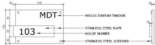
DETAIL SIGNAGE N.T.S
