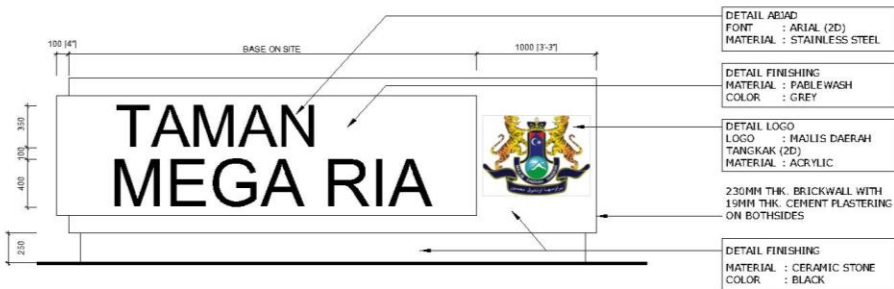
FRONT ELEVATION N.T.S
